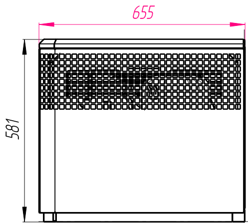
Вид справа Масштаб: 1:12
