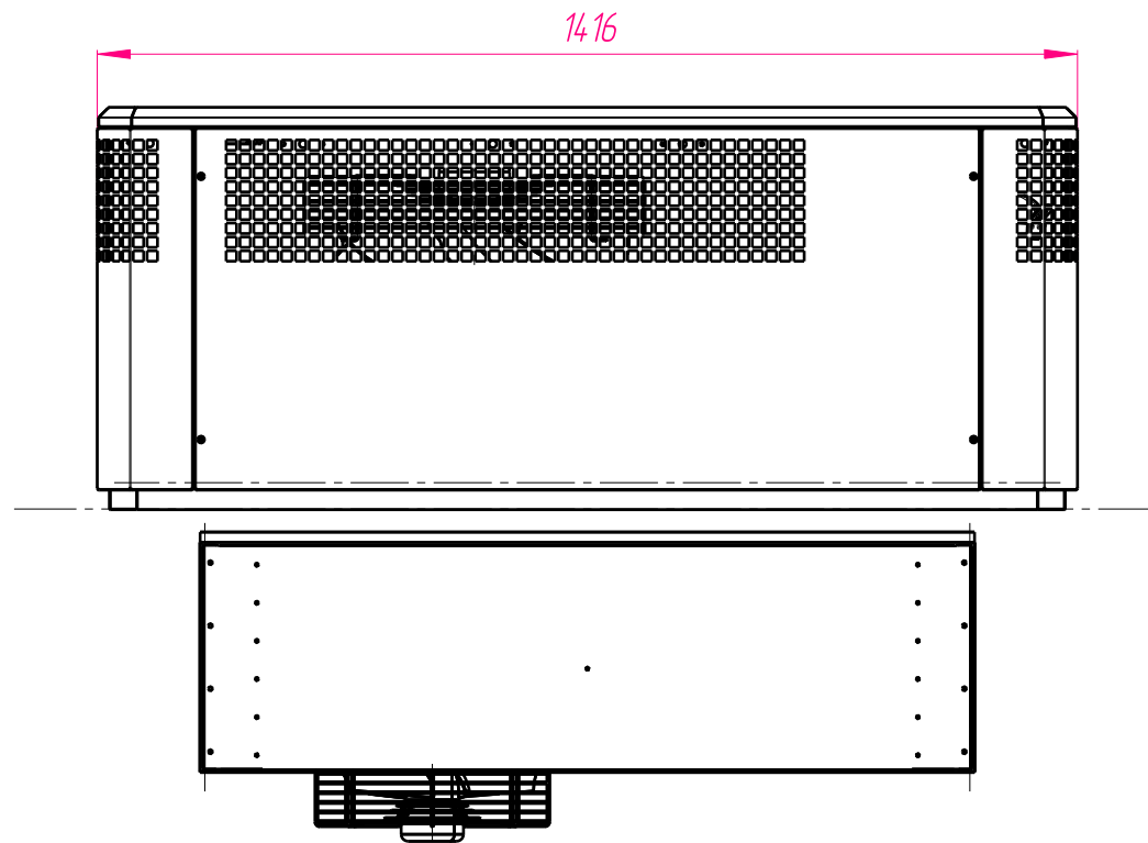
Вид спереди Масштаб: 1:12
